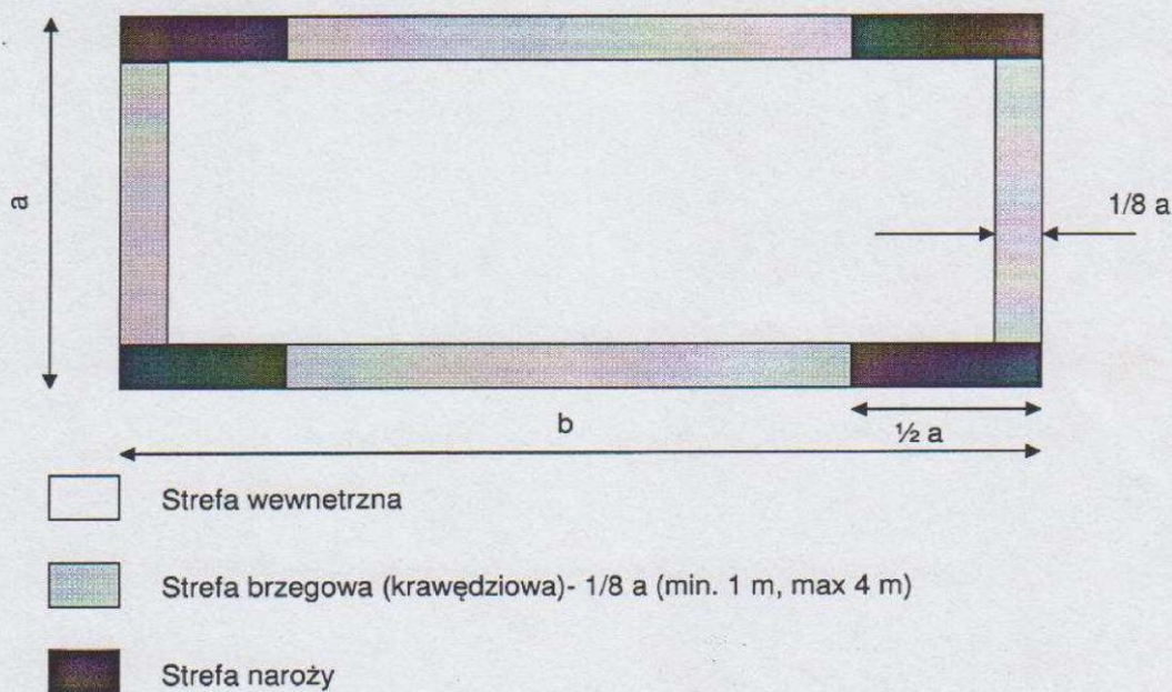
Rys. 2 Strefy w dachu płaskim w przypadku 1,5 a < b (rzut dachu zbliżony do prostokąta)
